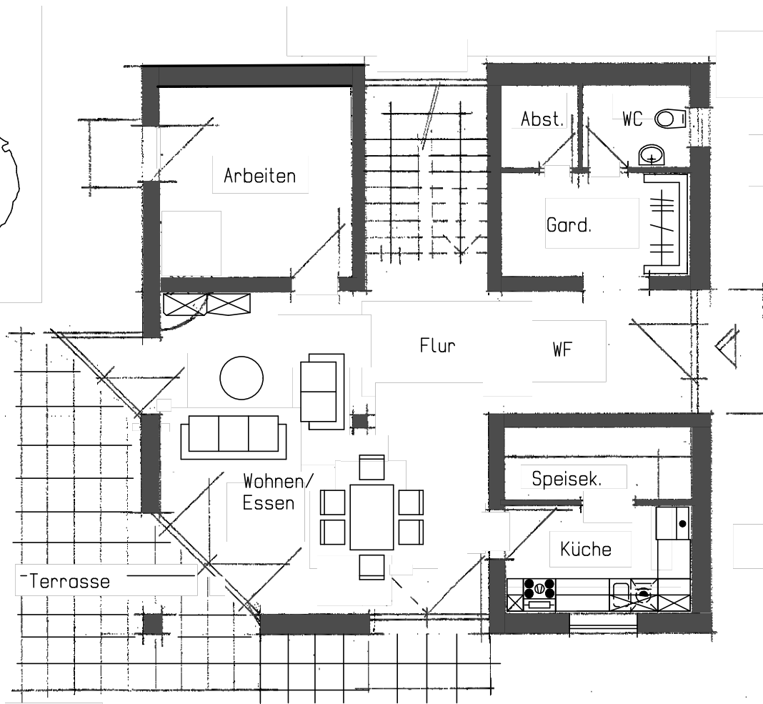
ERDGESCHOSS
